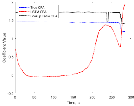
a.) Longitudinal Force Coefficient
